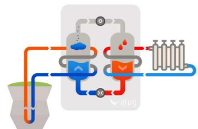
Boucle primaire – à gauche et boucle secondaire – à droite (source : AFPG)
